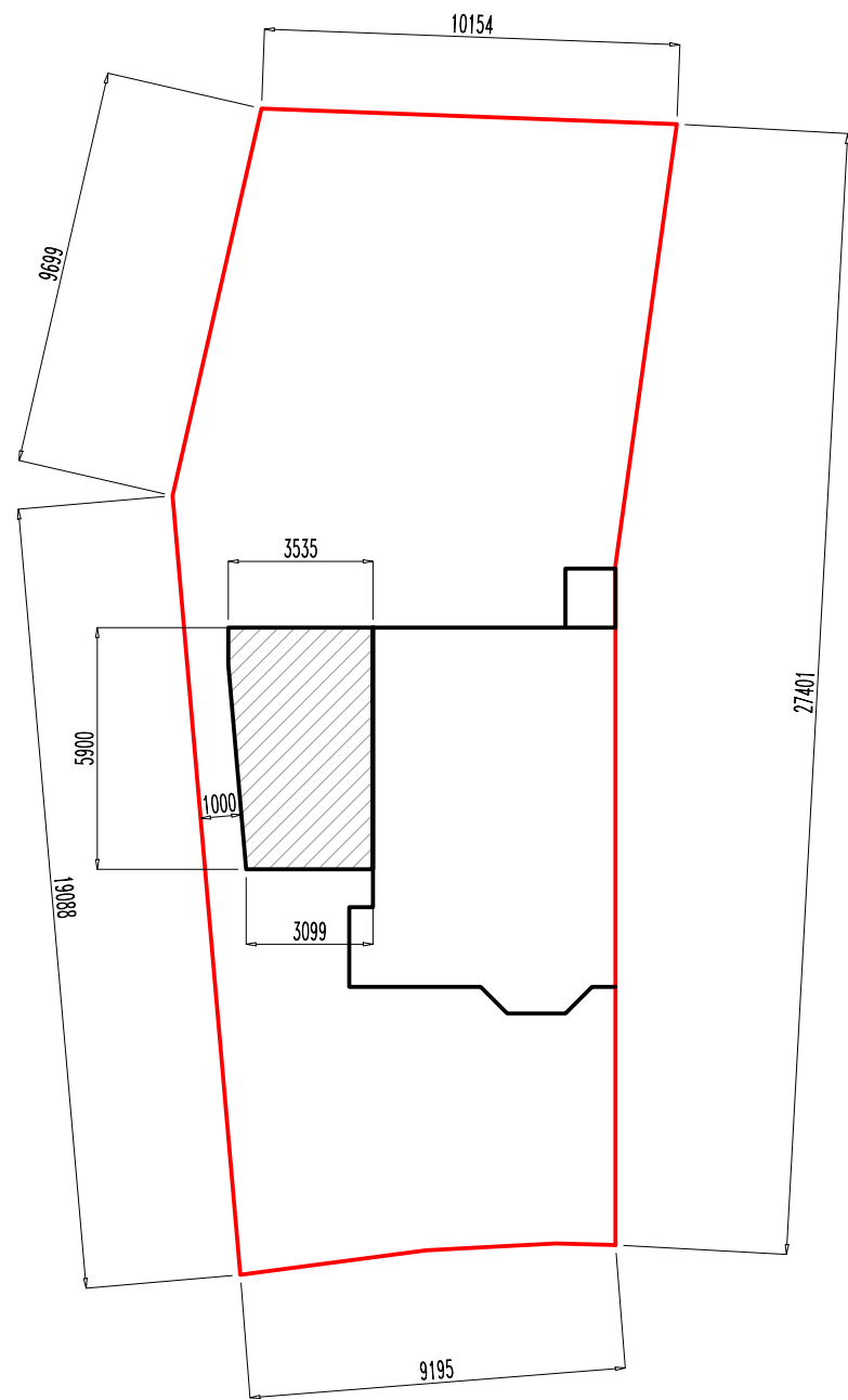
SITE PLAN 1:200
