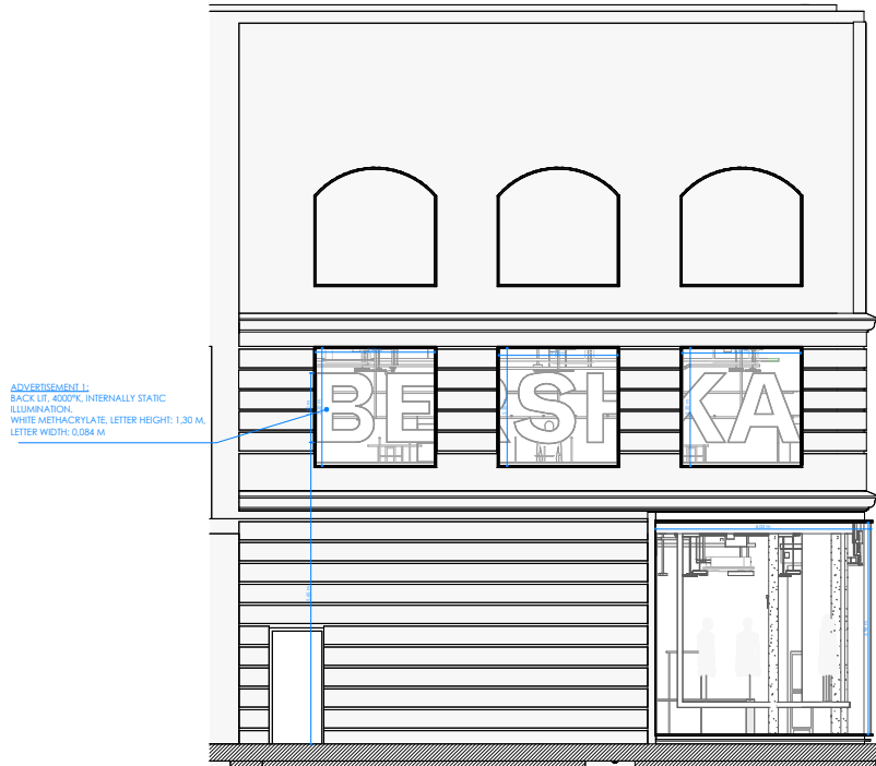
IMG_SEC_SHT_Fachada Calle-Street Façade 1 1 : 50
