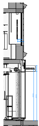
IMG_SEC_SHT_Fachada Calle-Street Façade 3 1 : 50
