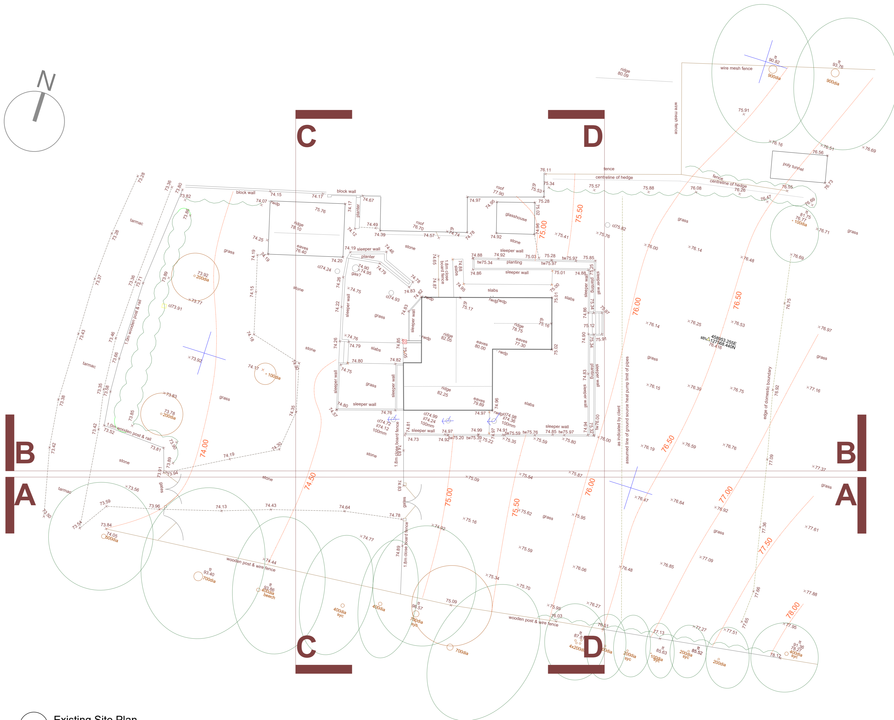
1 Existing Site Plan Scale: 1:200
