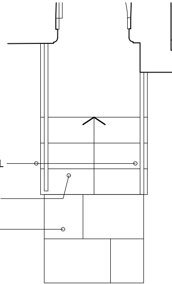
PLAN 1:50
