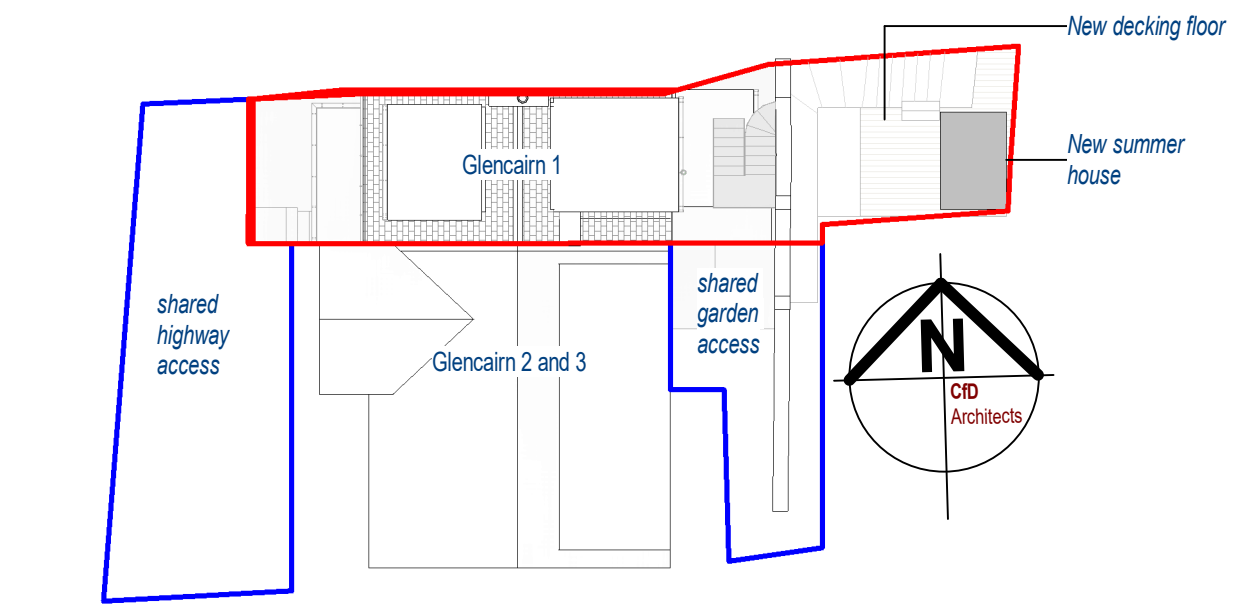
5 Site Plan 1 : 200
