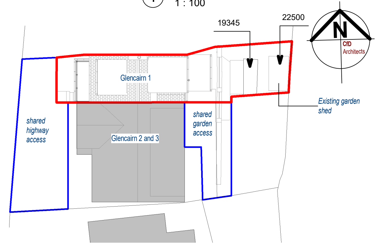
5 Site Plan 1 : 200
