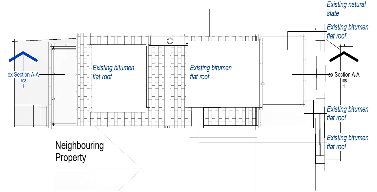
4 Roof Plan 1 : 100
