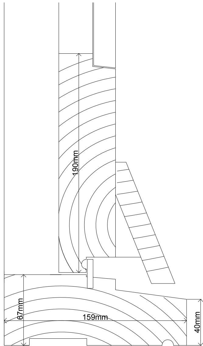
CILL
