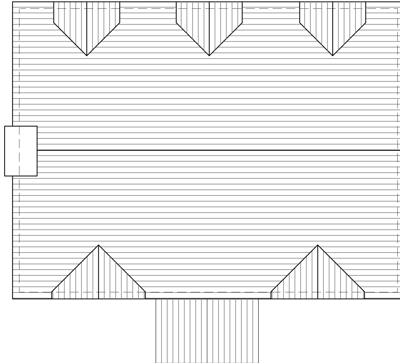
01 ROOF PLAN -- 1:50
