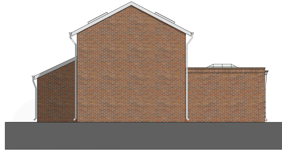
E2 Side Elevation 1:100
