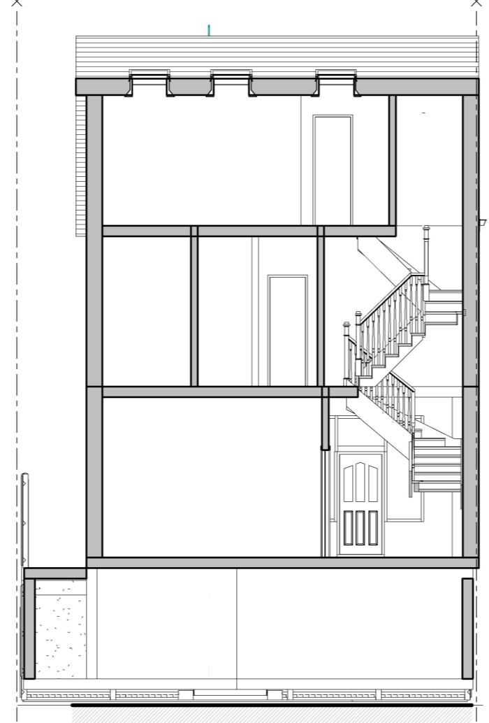
Section 2 1 : 100
