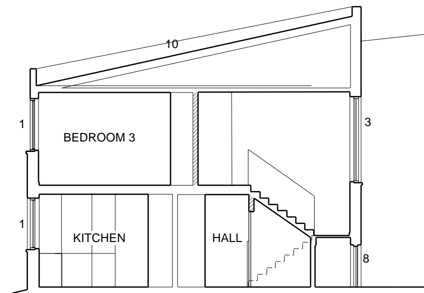
2 SECTION B.B Scale: 1:100
