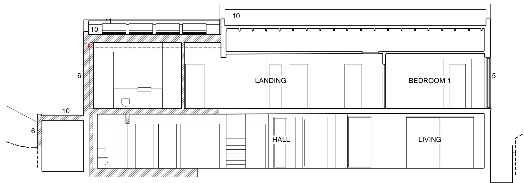
1 SECTION A.A Scale: 1:100
