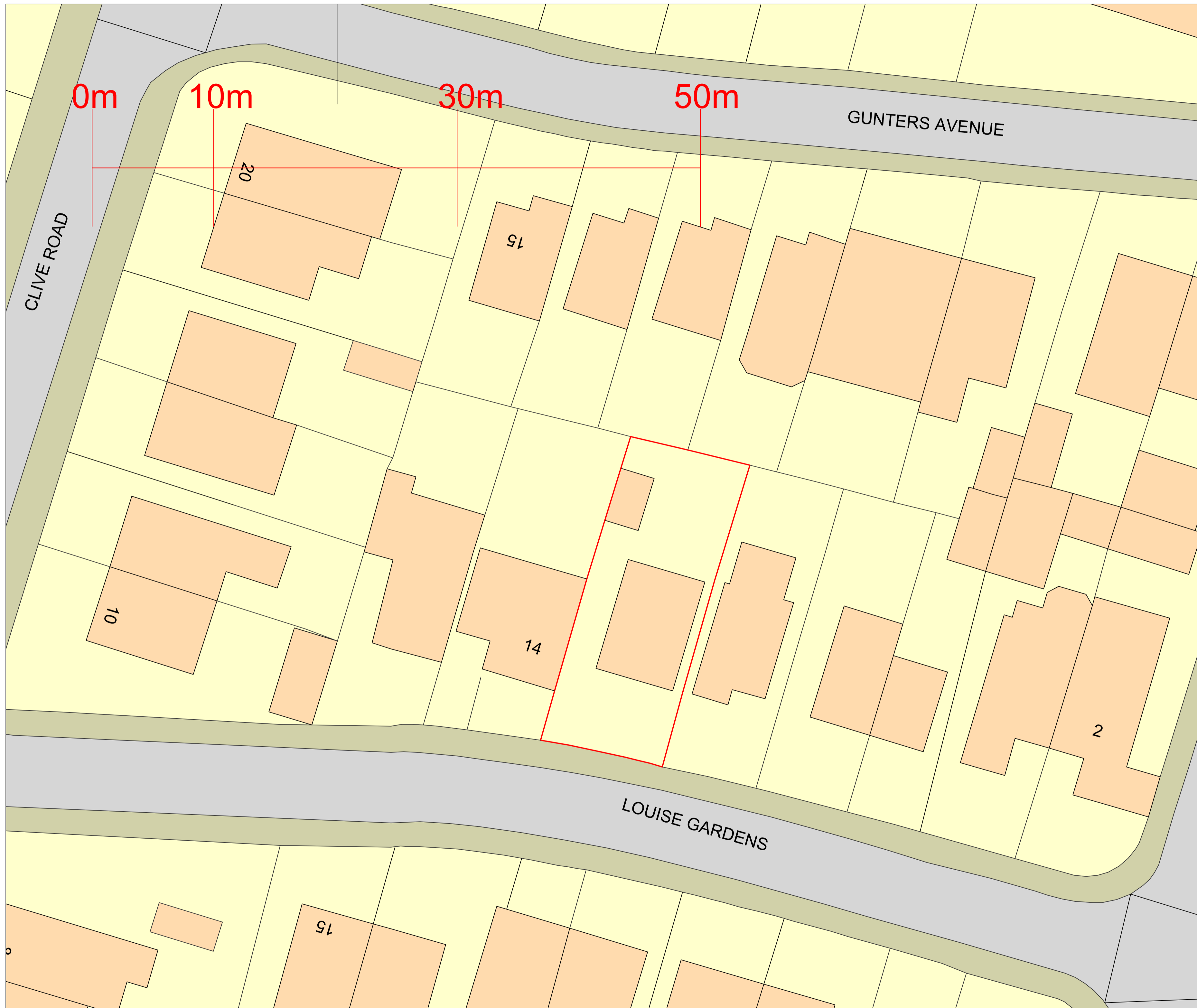
Site Plan 1:200
