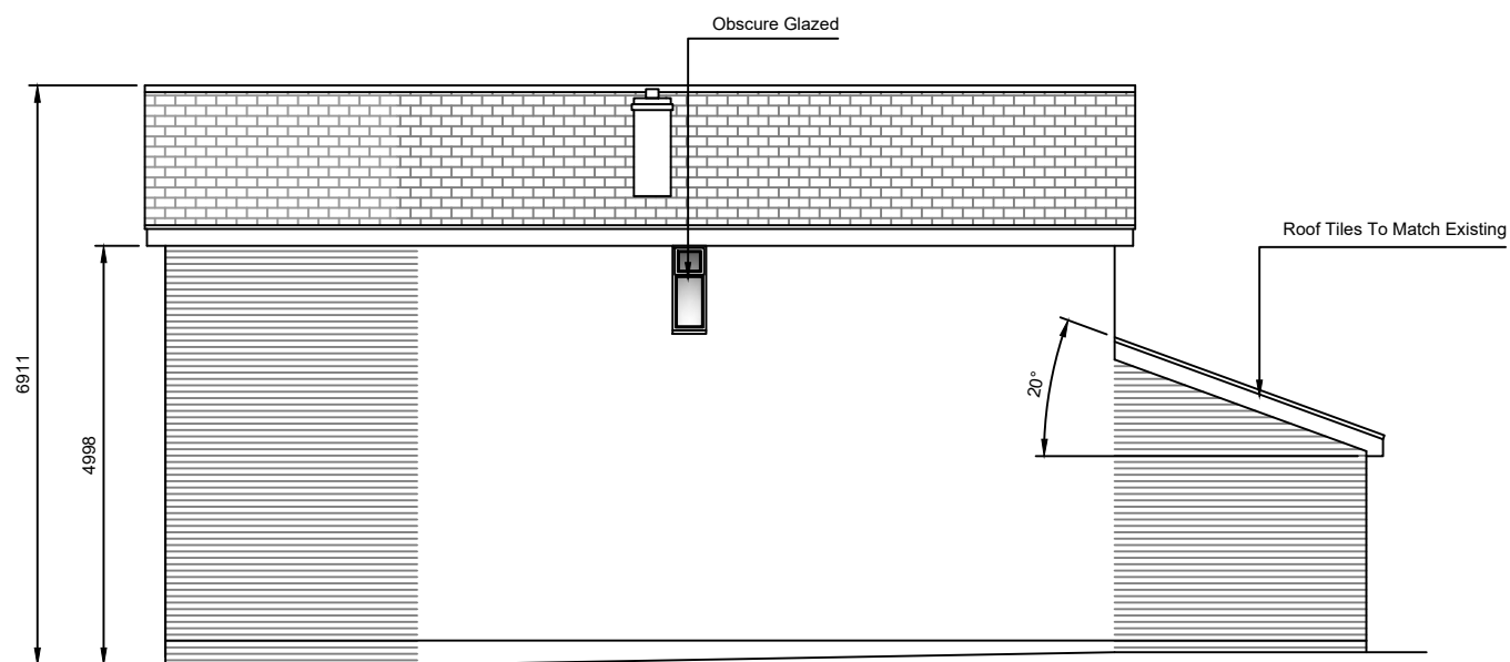
RIGHT ELEVATION
