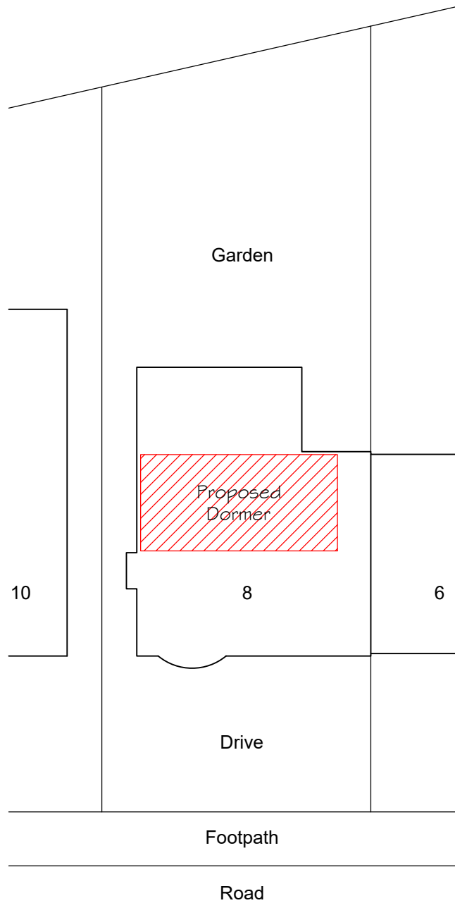
Site Plan 1:200
