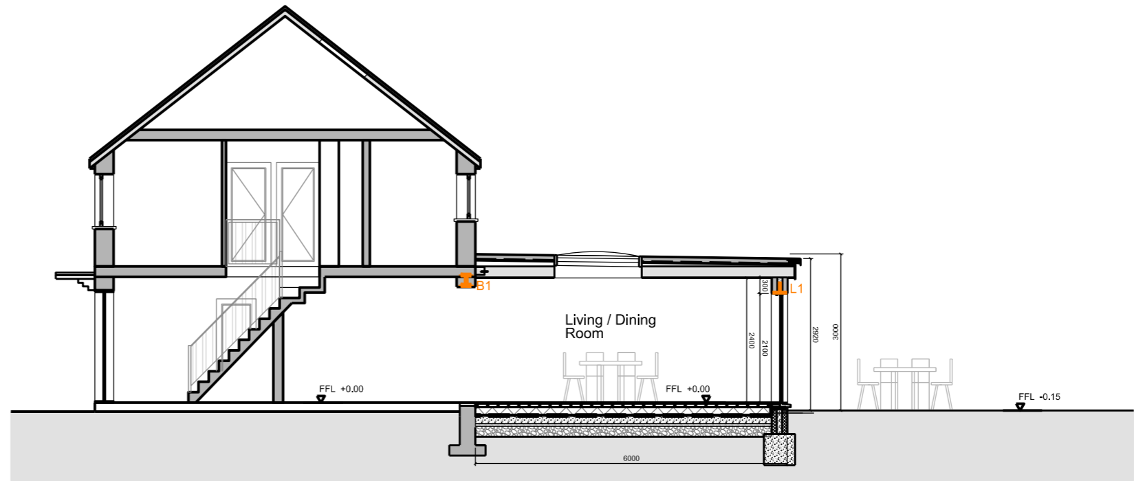
04 SECTION A-A 1:100
