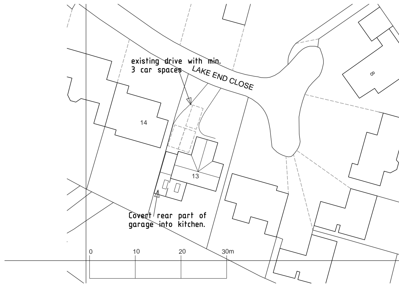
Site Plan 1 :500
