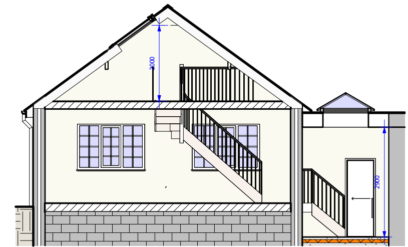
Annexe Stair Section 1 : 100
