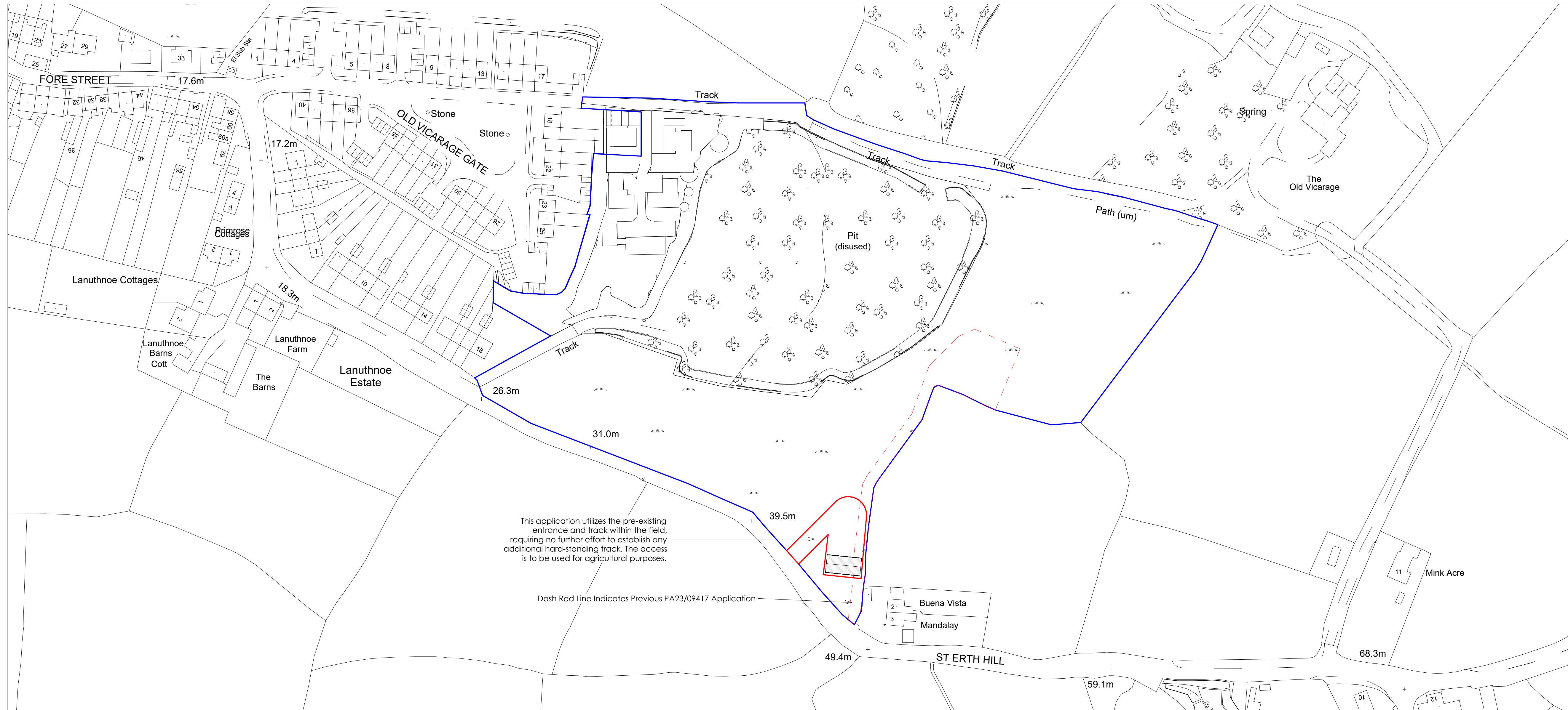
1 Site Boundary Plan 1 : 1000
