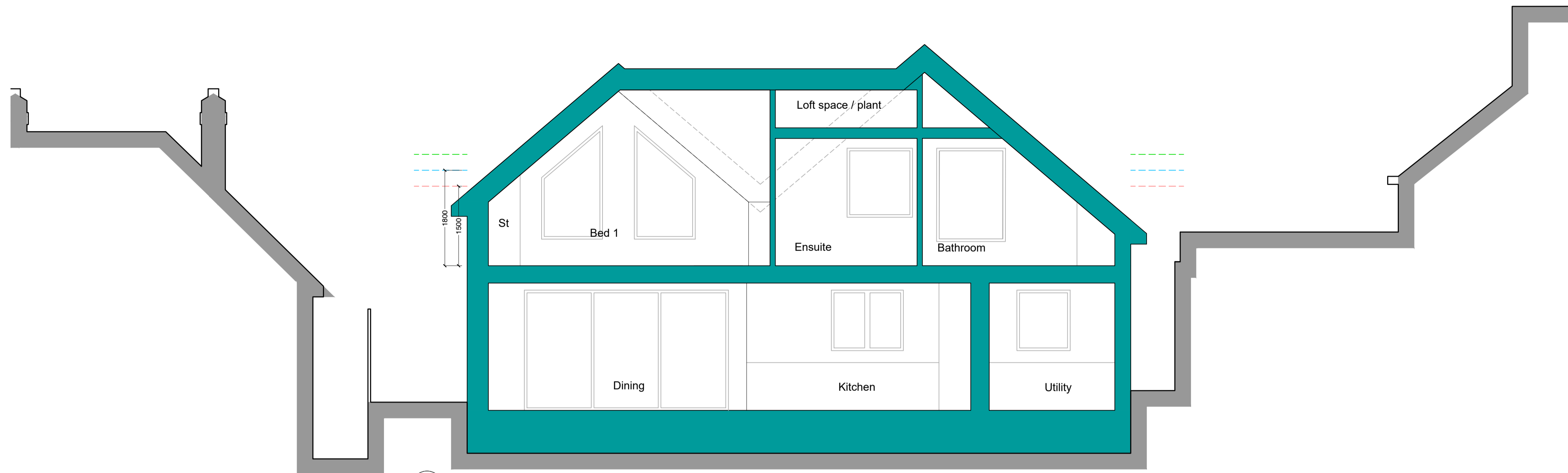
01 Section A - A Scale: 1:50
