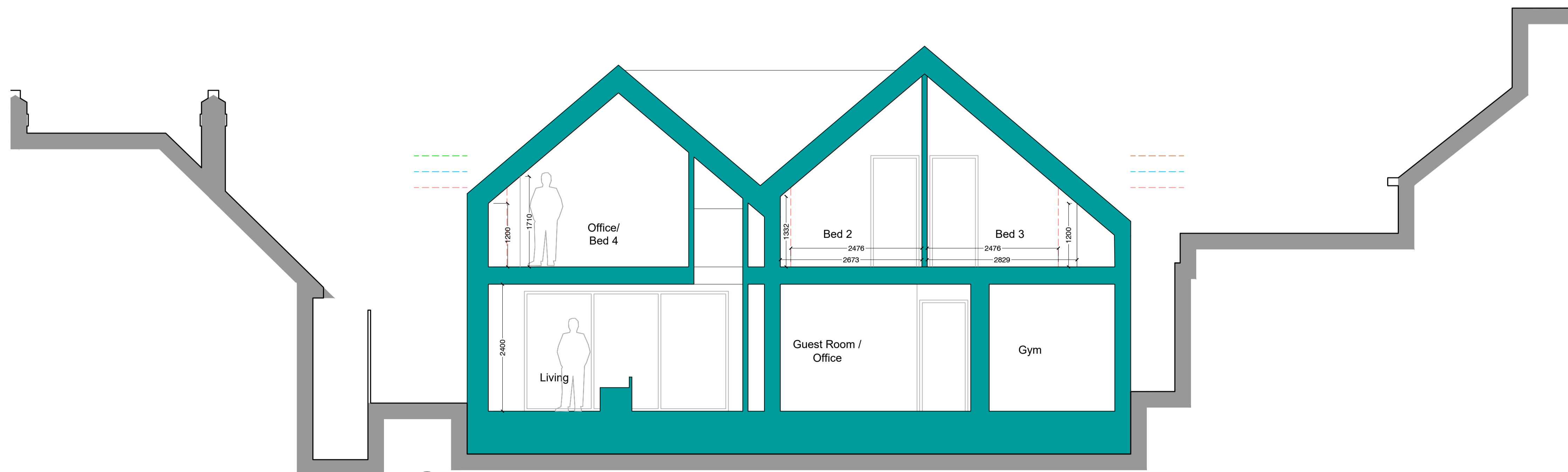
02 Section C - C Scale: 1:50
