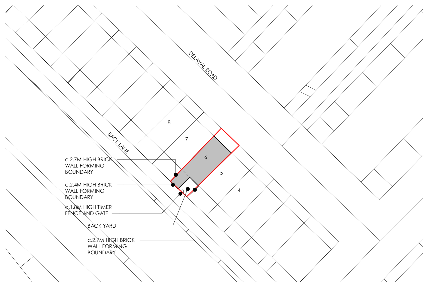
2 Site Plan_Existing 1 : 500
