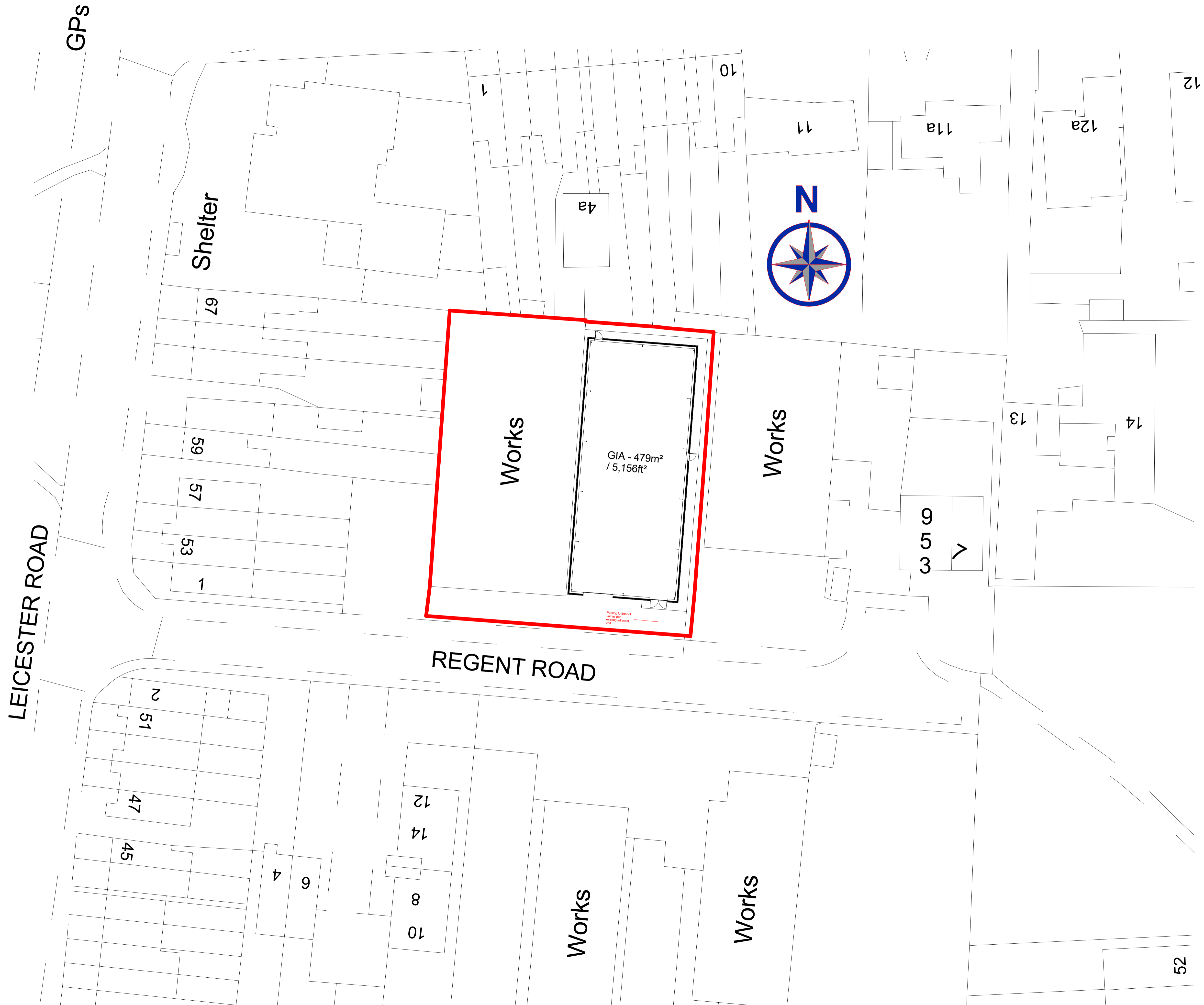
1 Site Layout Plan 1 : 250
