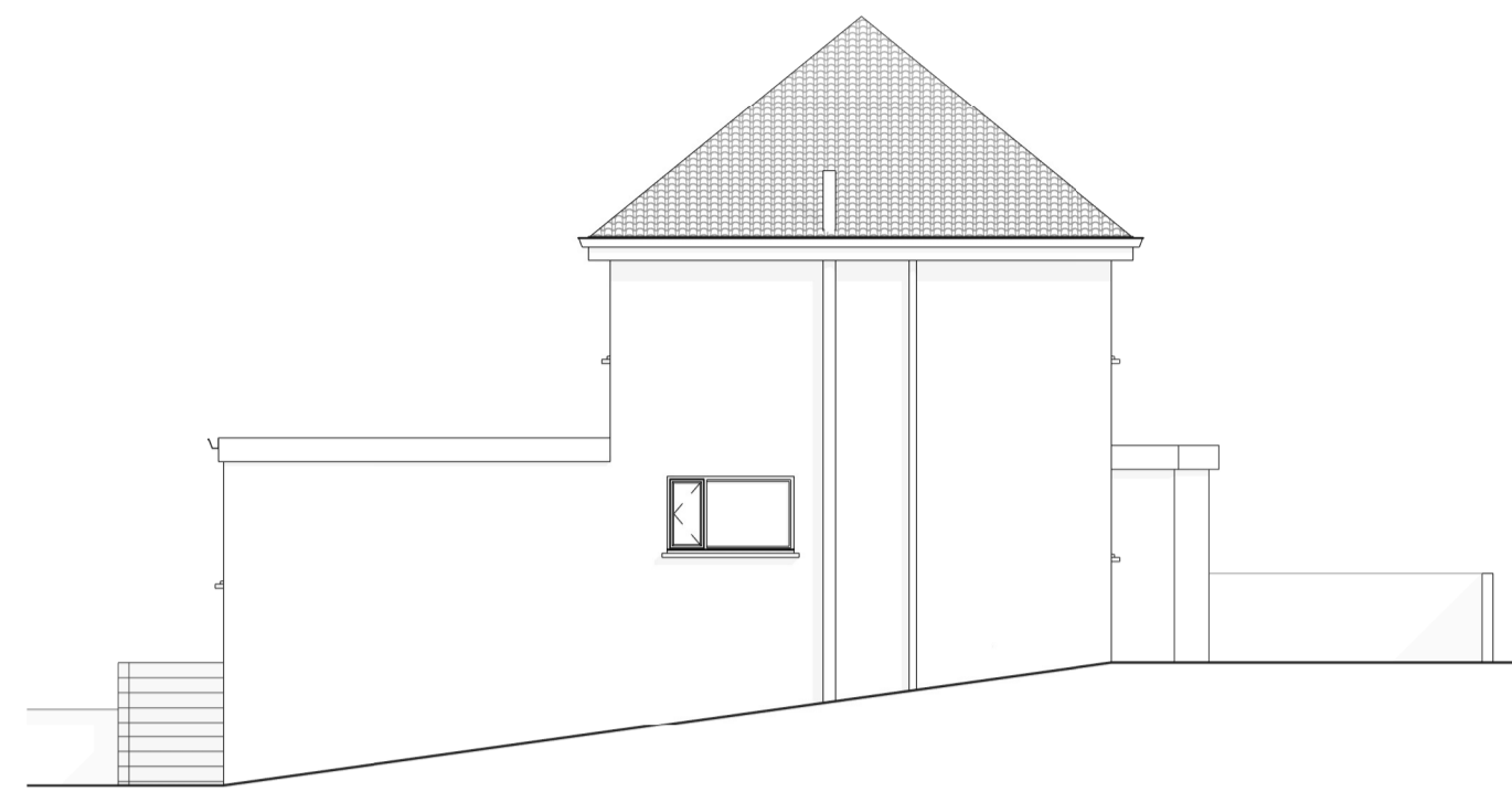
2 WEST ELEVATION SCALE: 1 : 100
