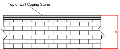
Brick wall 900mm high N.T.S
