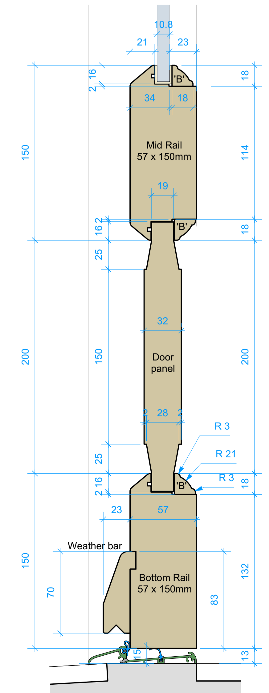
DOOR SECTION
