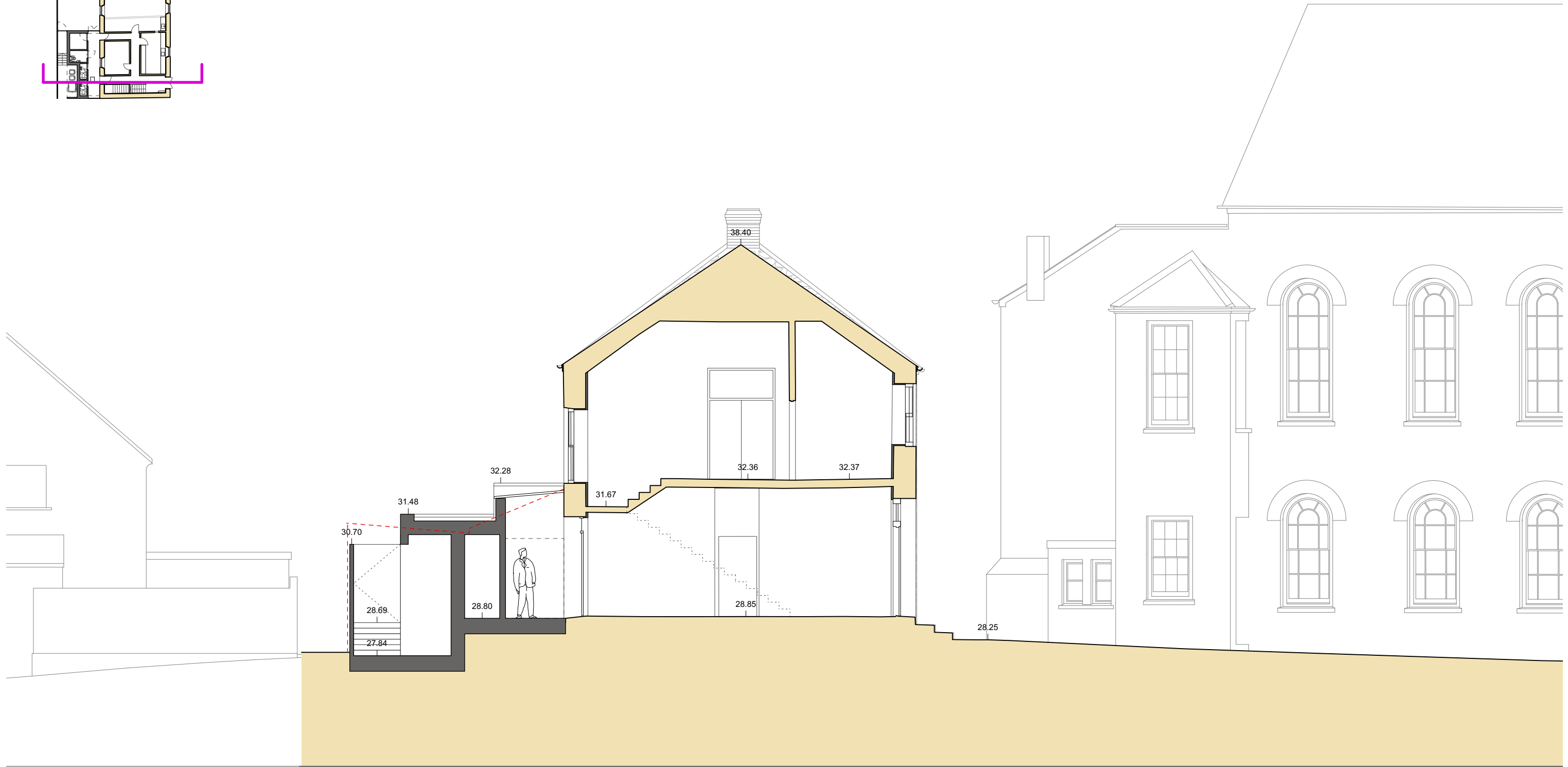
1 Cross section Scale: 1:100
