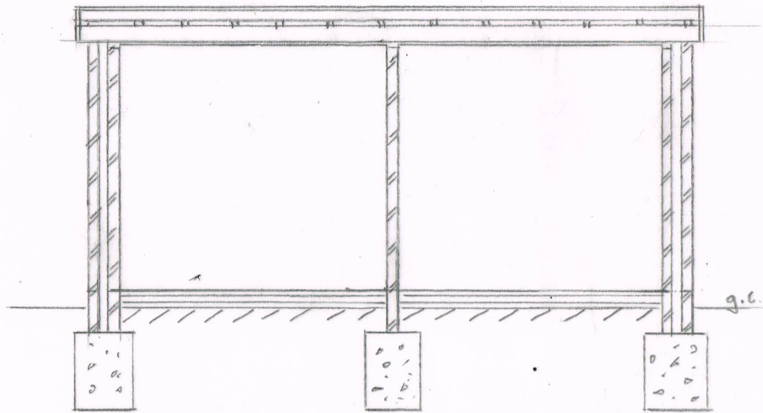
SECTION A-A 1/50
