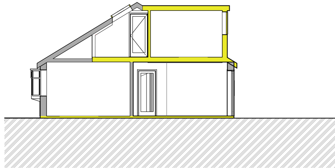
SECTION A:A
