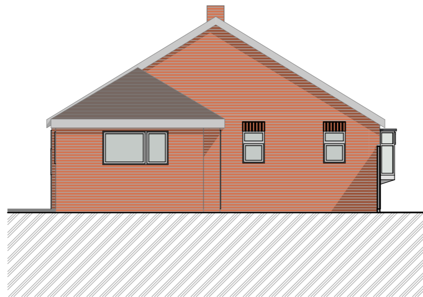
FLANK ELEVATION
