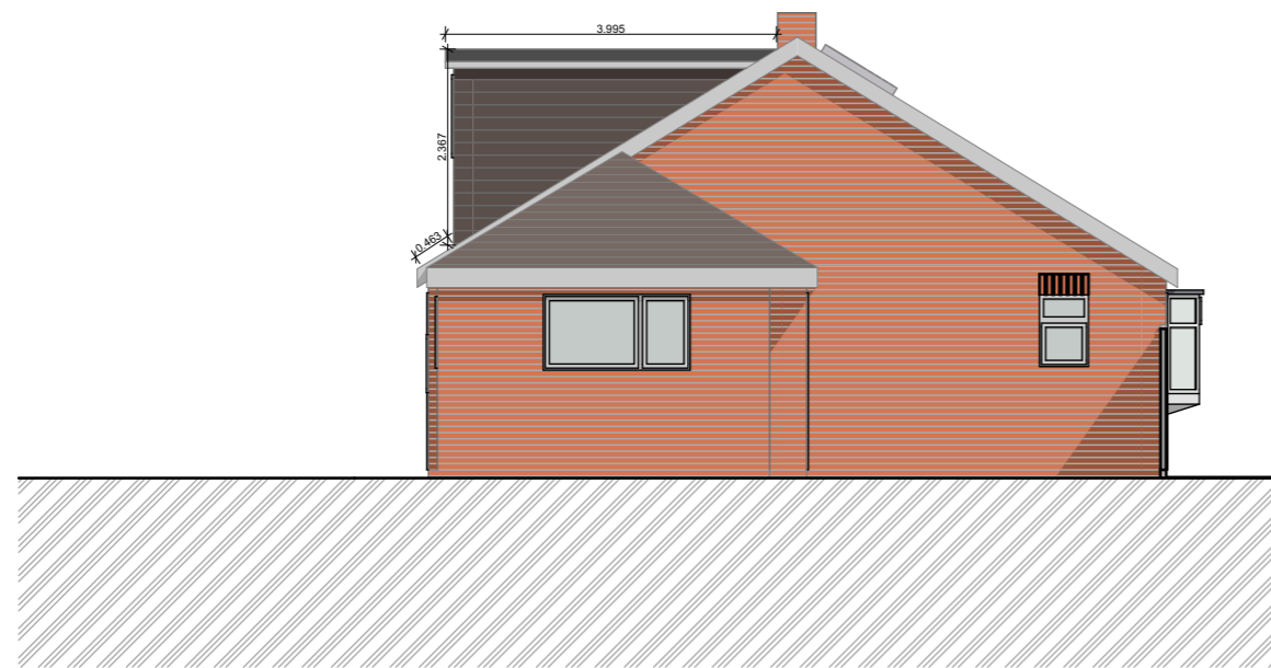
FLANK ELEVATION
