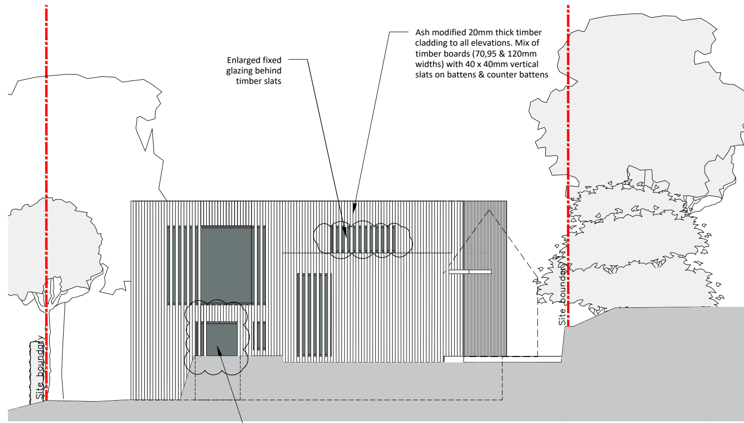
01 201 Elevation 02 1:100
