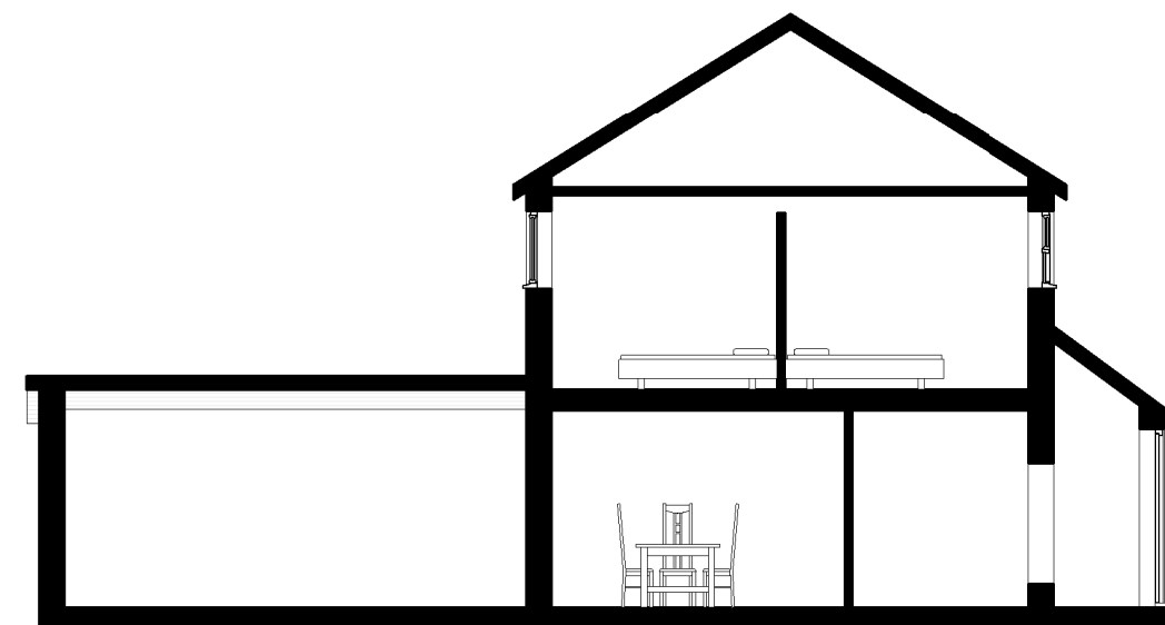
5 Section 1 1 : 100
