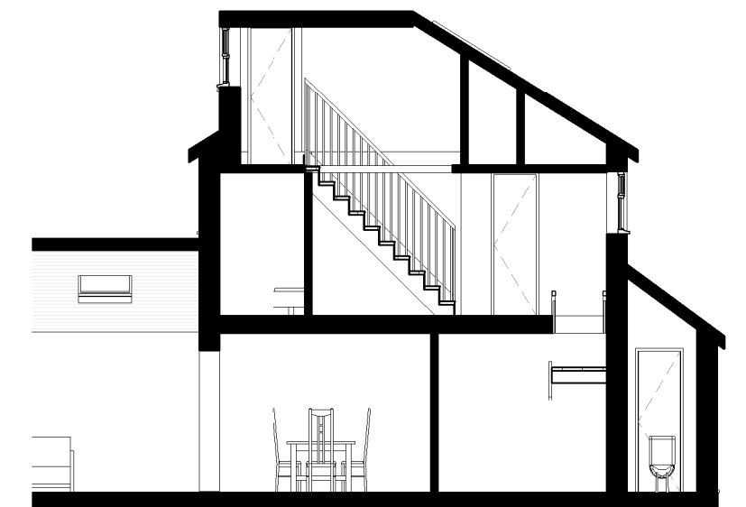
6 P- Section 2 1 : 100
