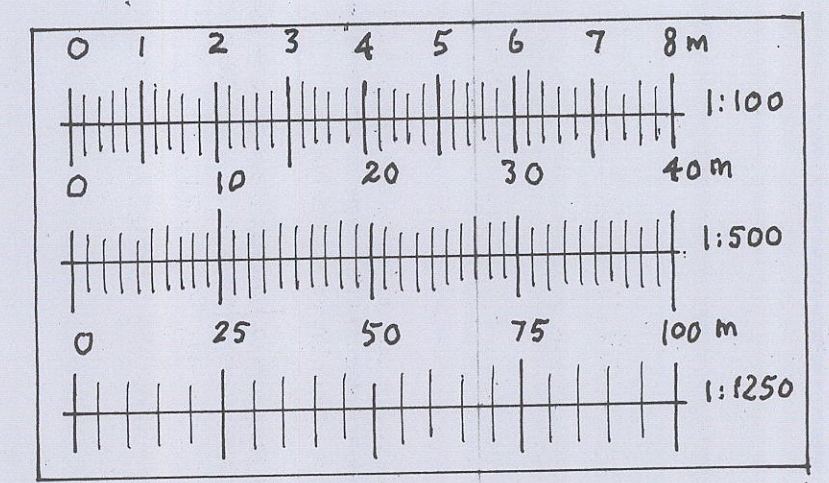
BAR SCALES
