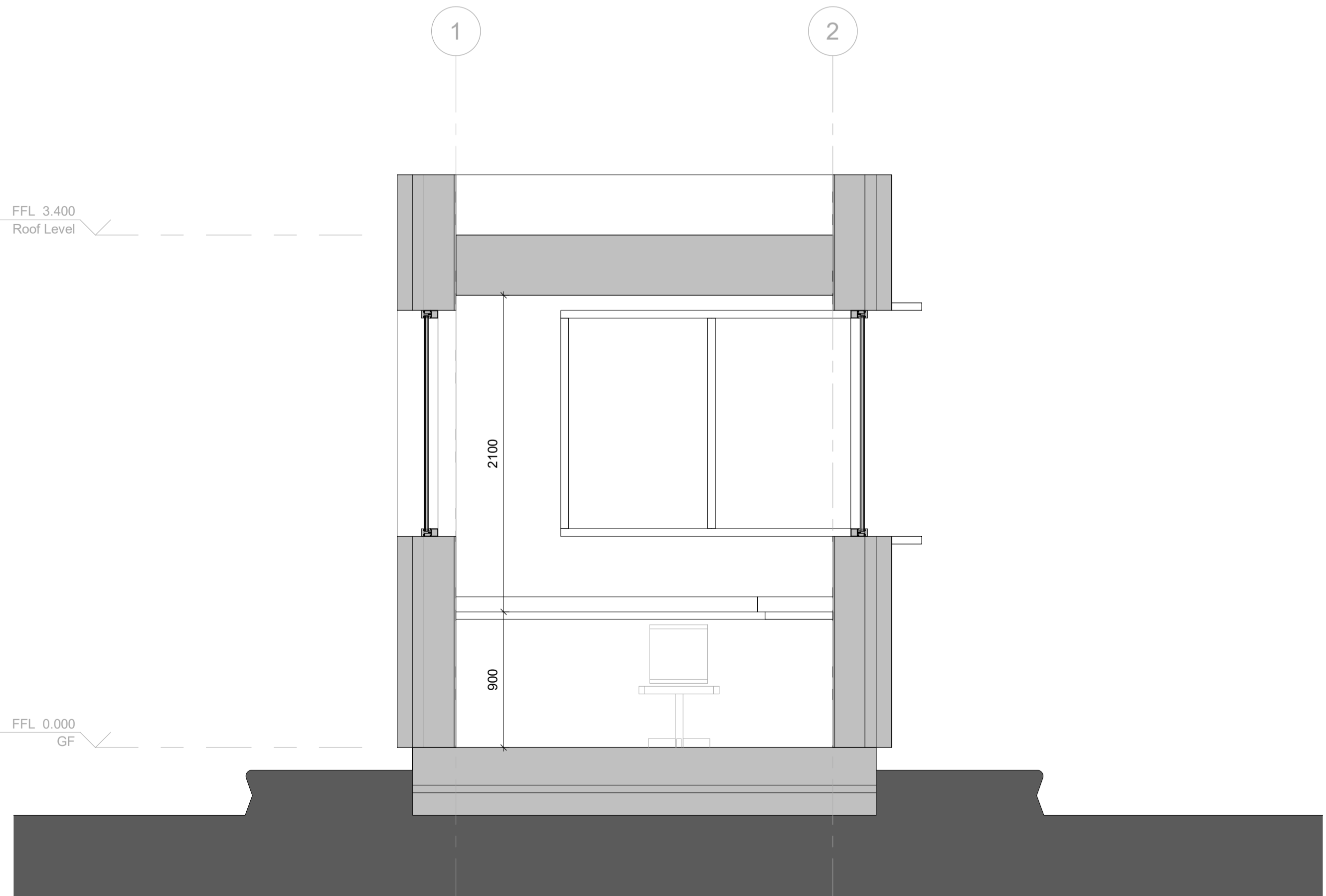
2 Section 2 1 : 25
