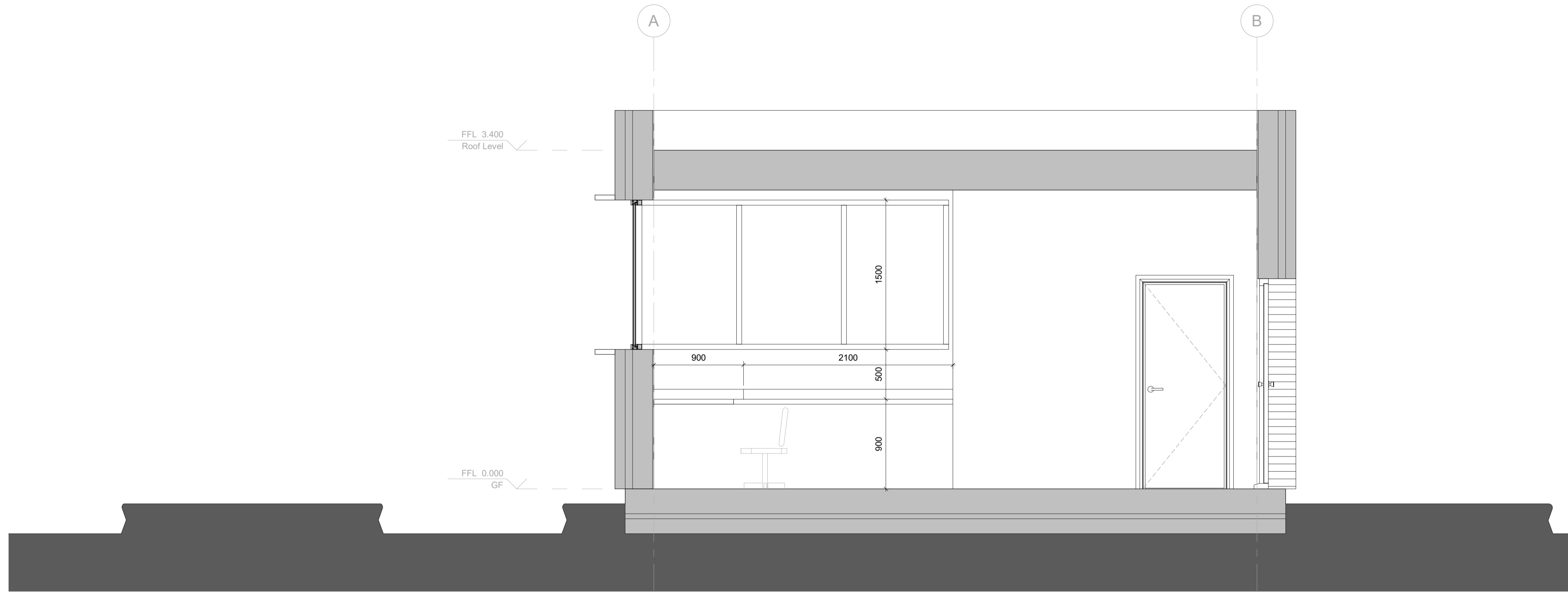
1 Section 1 1 : 25
