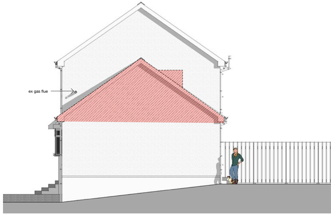
E :: EXISTING SIDE ELEVATION 2 scale: 1:100
