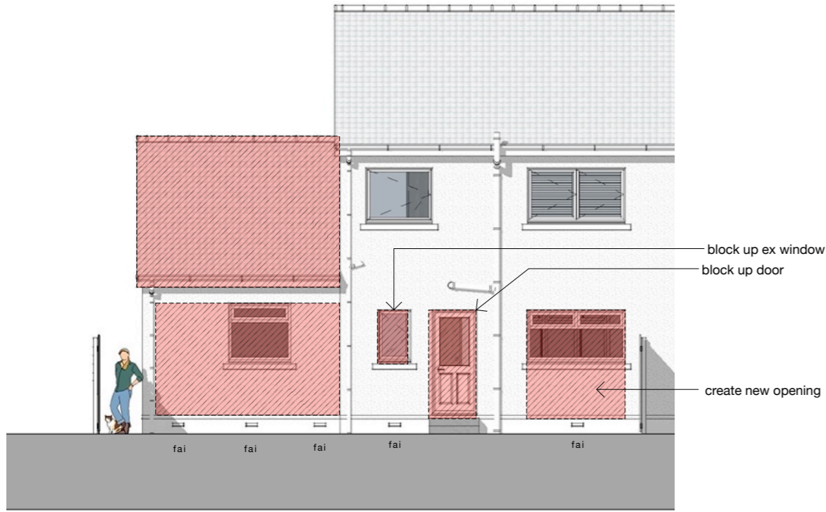
E :: EXISTING REAR ELEVATION 1 scale: 1:100
