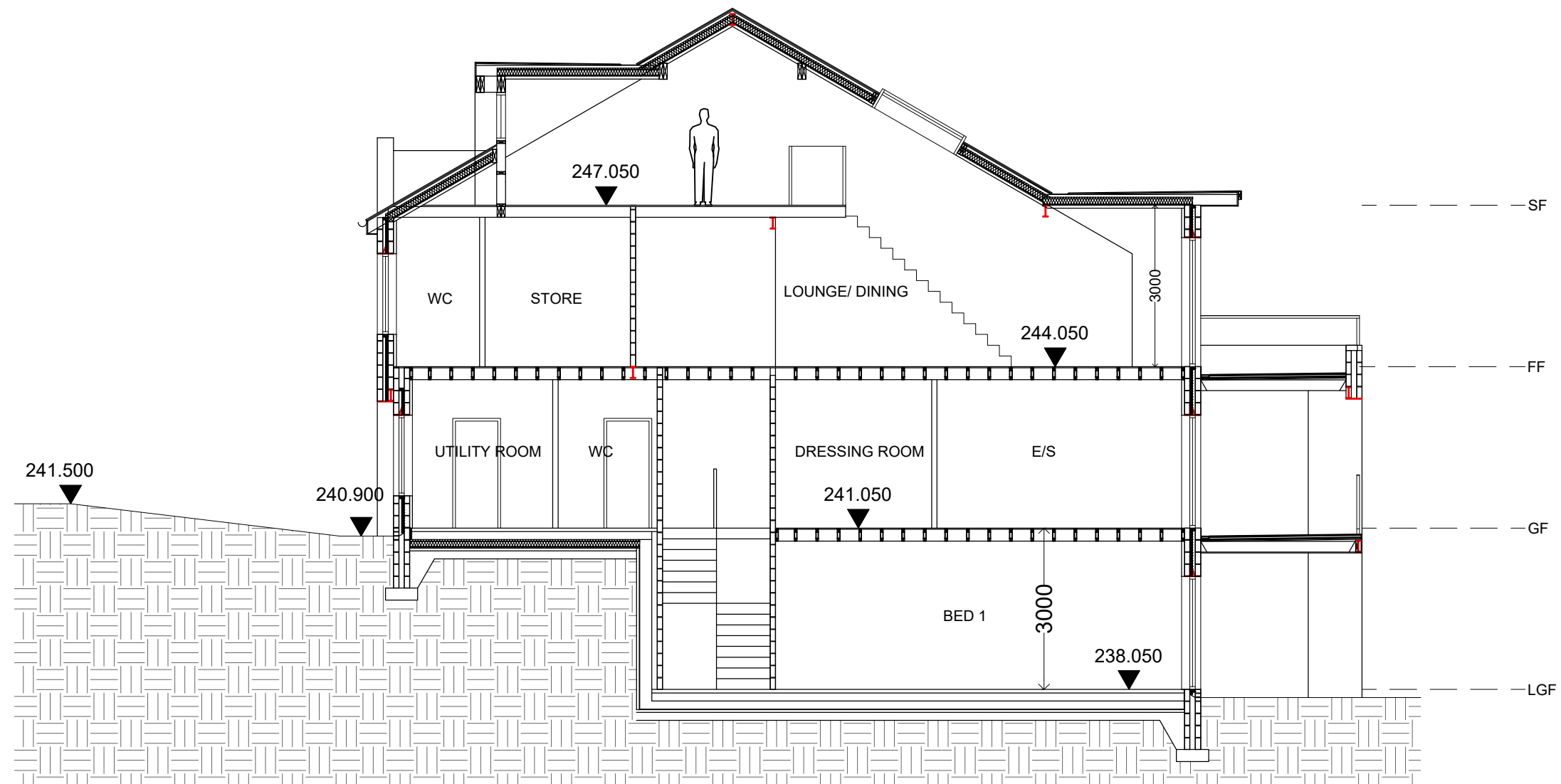
SECTION A-A
