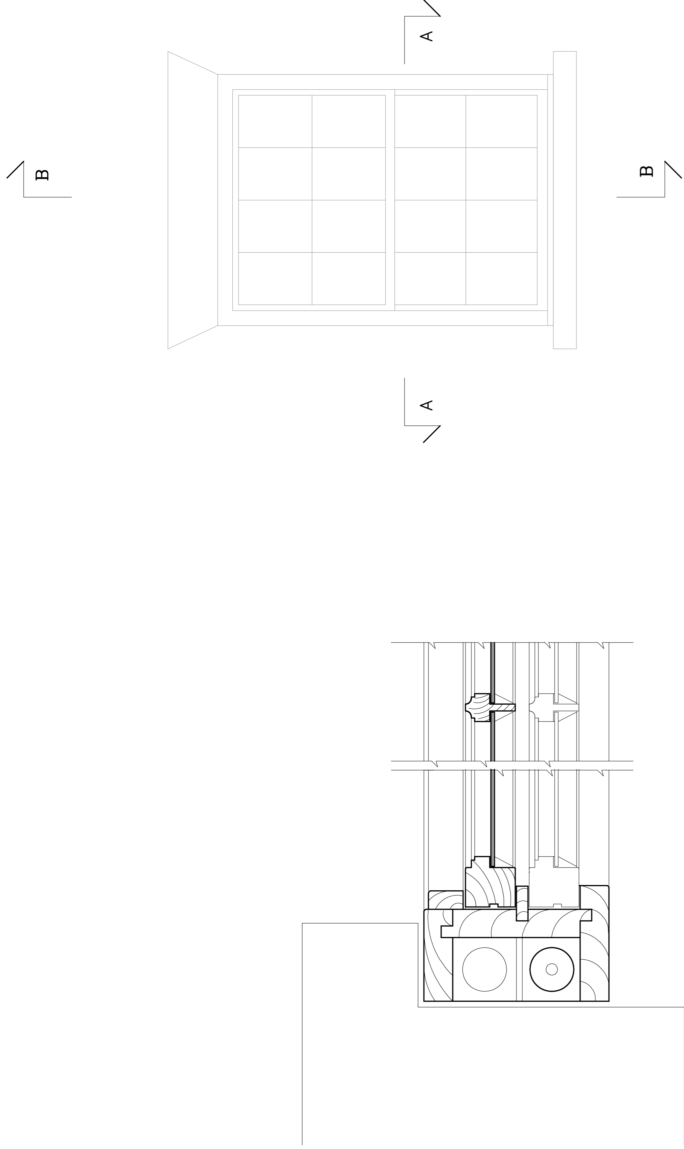
SECTION A-A Scale 1:2
