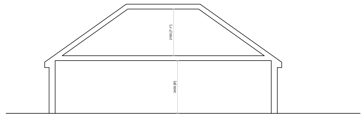
EXISTING SECTION 1 : 100
