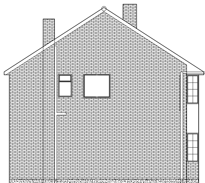
LEFT FLANK ELEVATION
