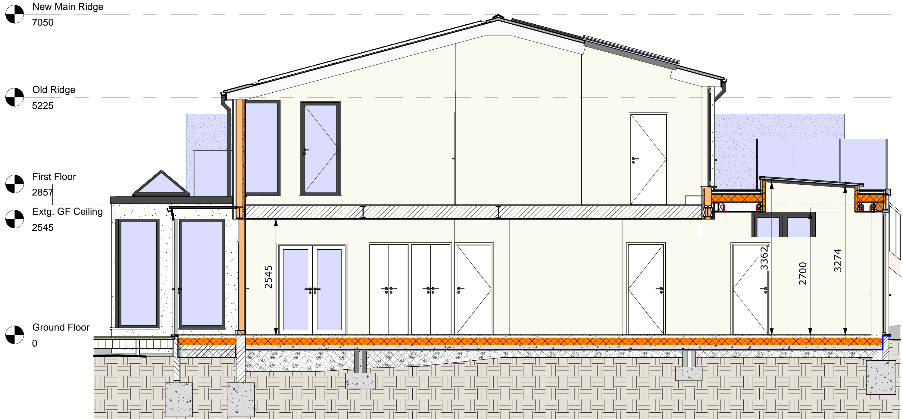
Section A-A 1 : 50
