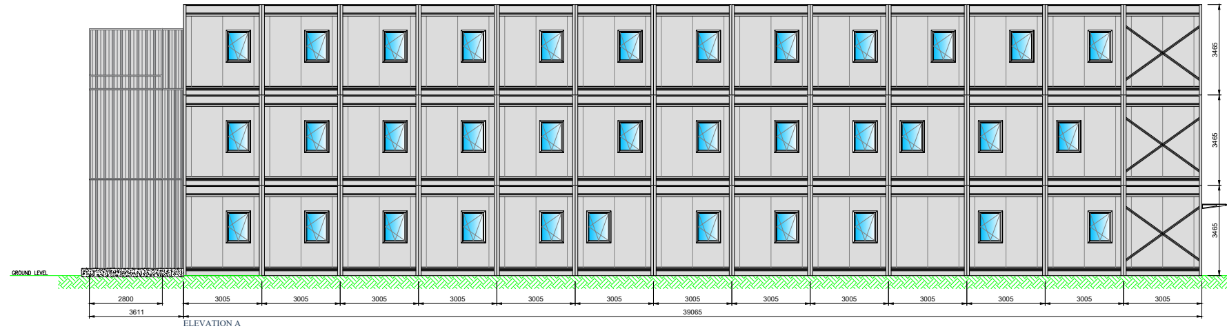
ELEVATION A
