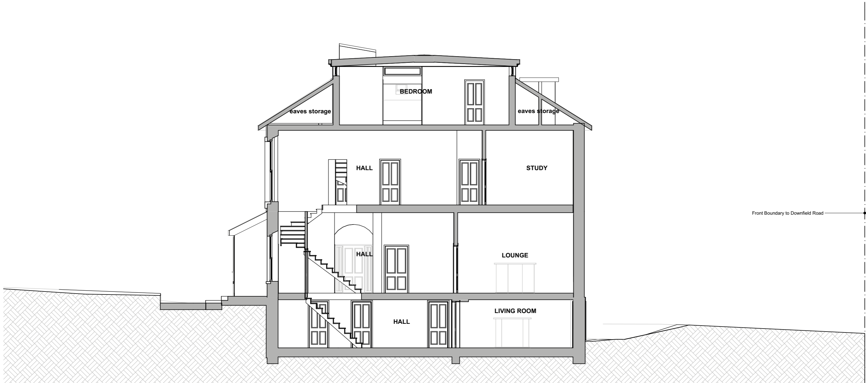
1 Section BB 1:100
