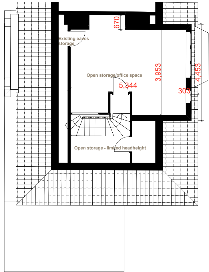
Loft plan
