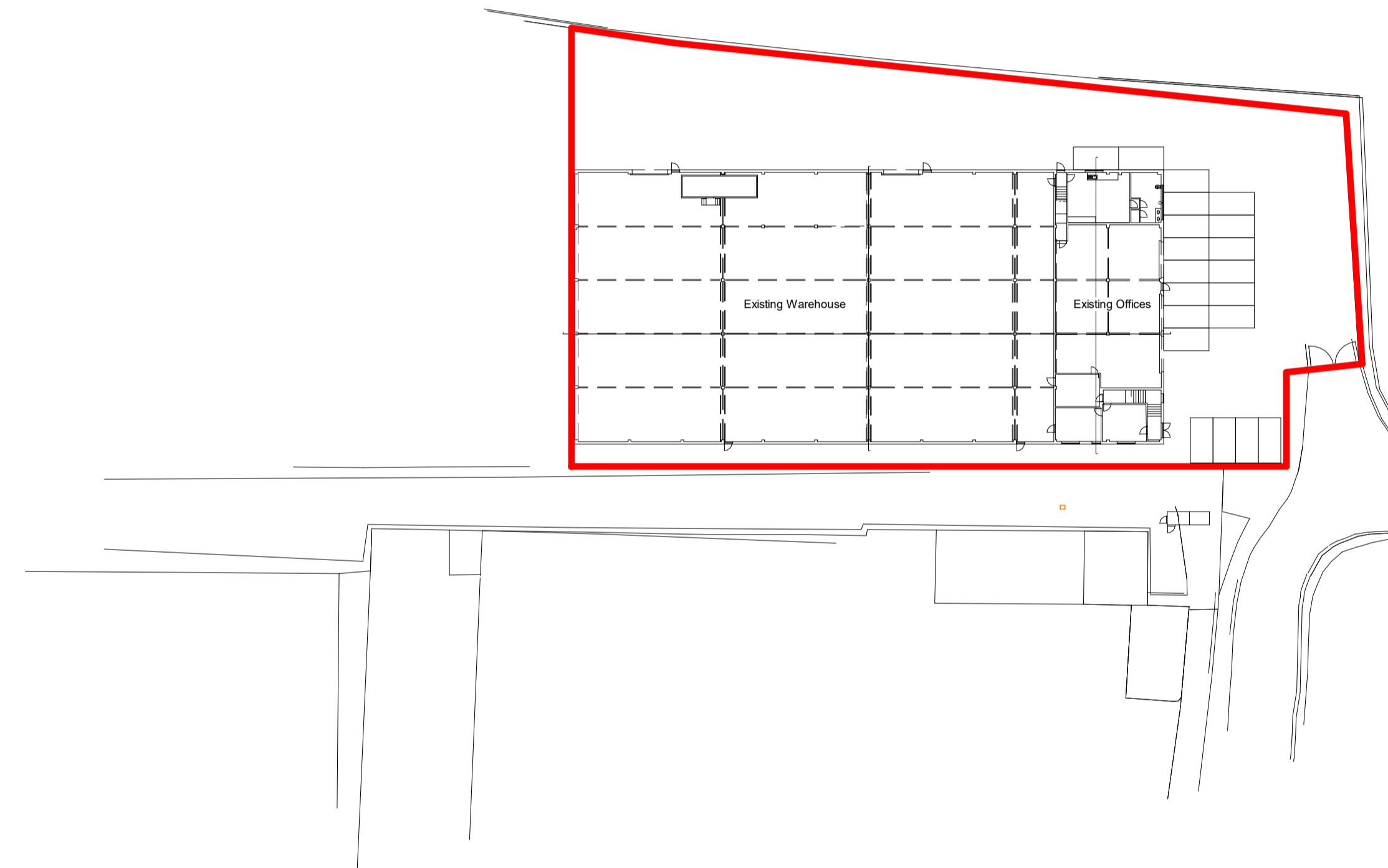
1 Existing Site Plan 0008 1 : 500
