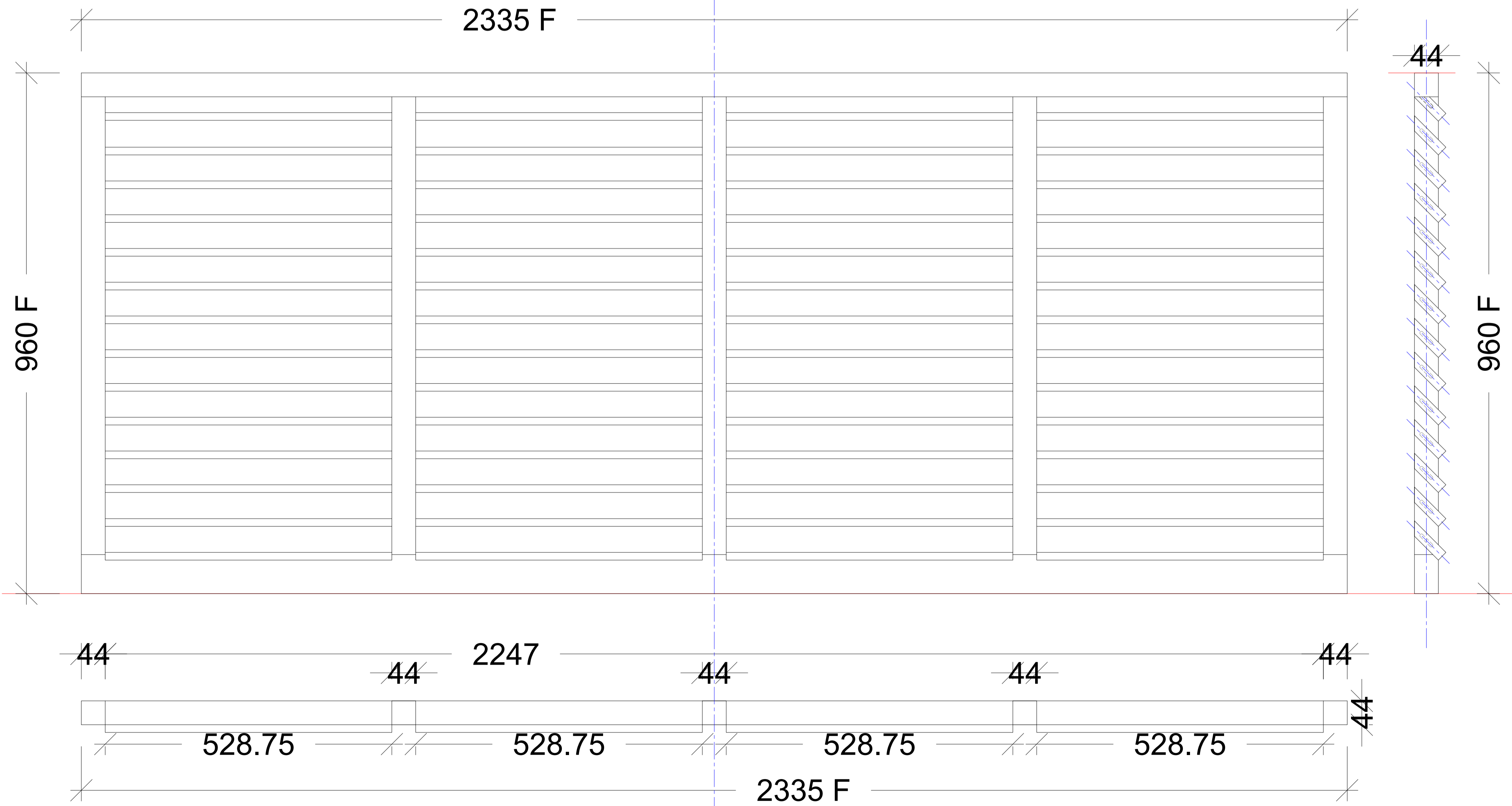
1 ELEVATION Scale: 1:5
