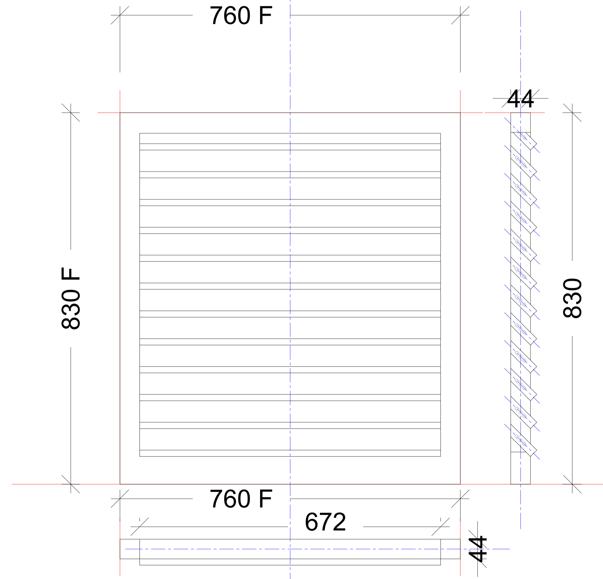
1 ELEVATION Scale: 1:5
