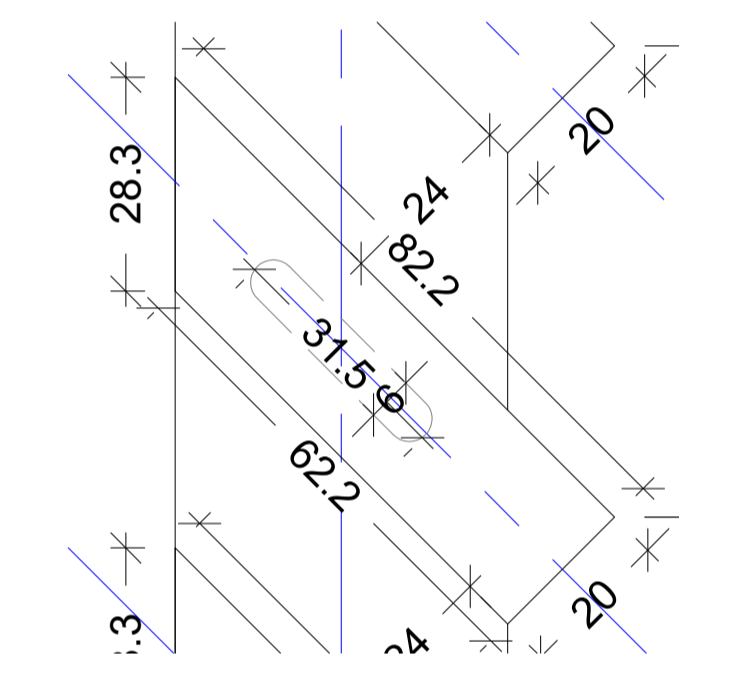
4 LOUVRE Scale: 1:1
