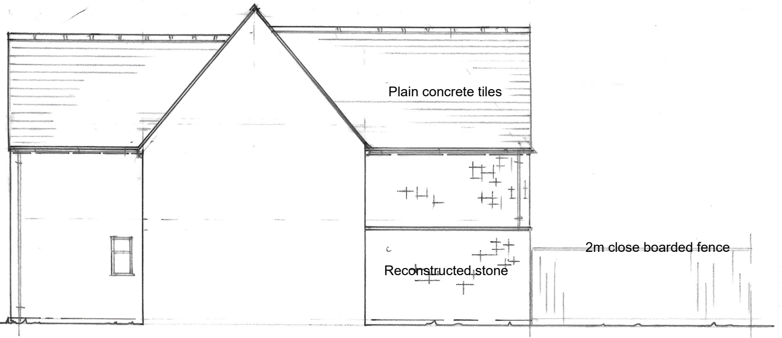
SW ELEVATION
