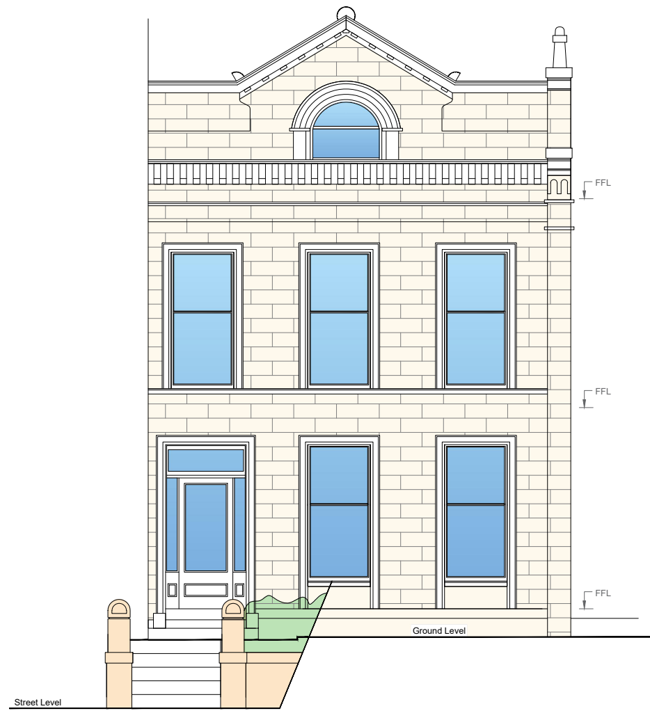
Front Elevation Scale: 1/100 @ A3
