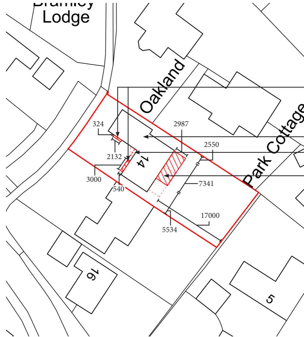
SITE PLAN 1:500
